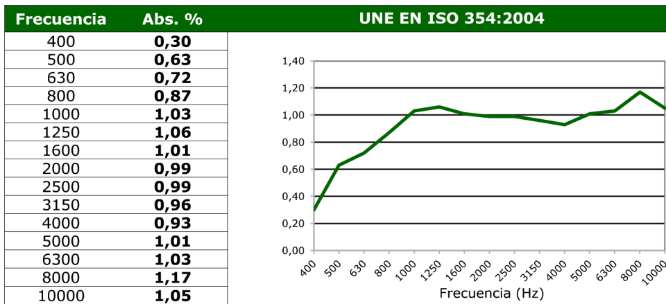
Absorción acústica en cabina alpha
